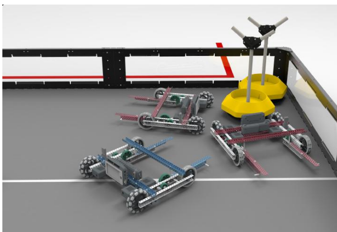
图 12b 红方联队的 2 台机器人正 在囤积环塔
